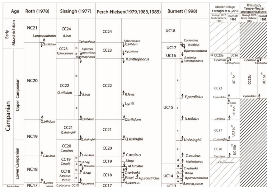
شکل ۹: نانوفسیل‌های آهکی شاخص و محل قرارگیری آنها در بایوزون‌های مربوطه و الگوهای جهانی استاندارد بازه زمانی زمین‌شناسی کامپانین در برش تنگ نیزار (برگرفته از فروغی و همکاران، ۱۳۹۱، با اندکی تغییرات).
