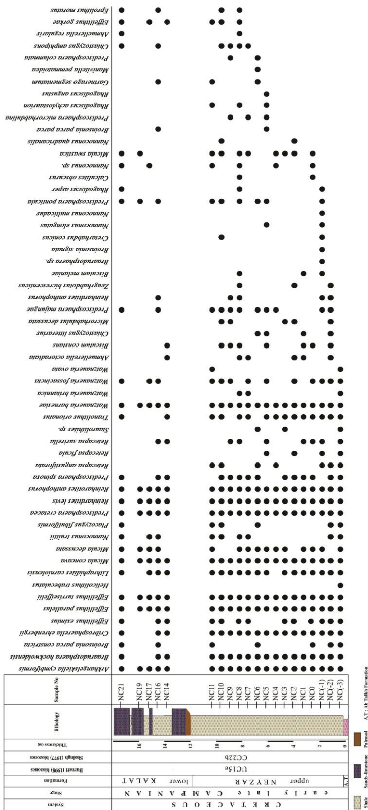
شکل ۴: گسترش و پراکندگی گونه‌های نانوفسیل‌های آهکی در برش تنگ نیزار
