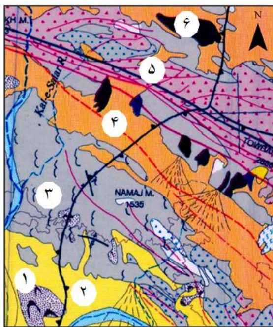
نقشه ژئومورفولوژی: ۱- تپه‌های شنی ۲- کفه‌های رسی ۳- بدلندها ۴- دشت‌های آبرفتی ۵- سنگهای آتشفشانی و دایک‌ها ۶- پادگانه‌های آبرفتی
