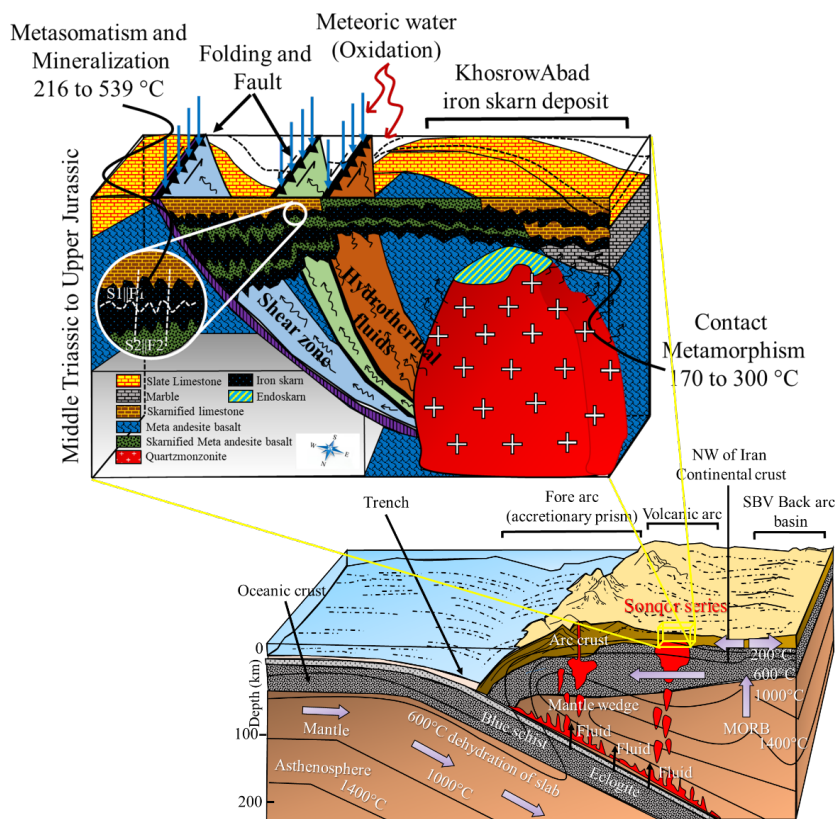
شکل ۱۴: محیط تکتونوماگمایی و مدل پیدایش کانسار اسکارن آهن خسروآباد
