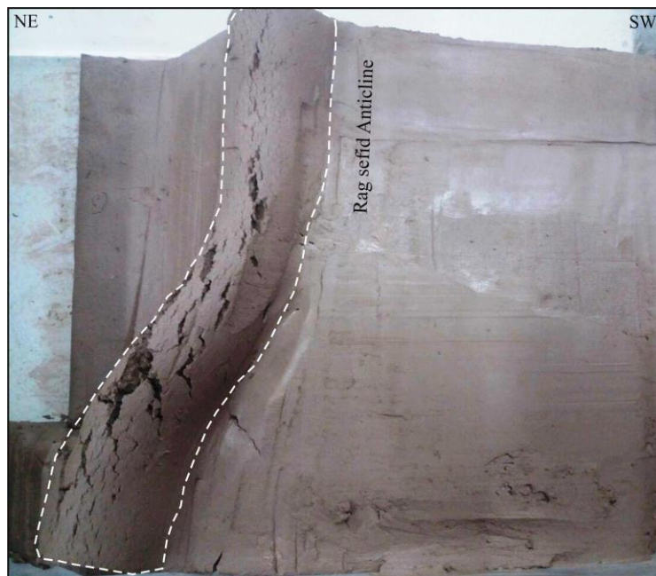
شکل ۱۲: تاثیر کاهش ضخامت نمک در مدل سازی که منجر به ایجاد تاقدیس با دامنه بیشتر و طول موج کمتر شده است.
