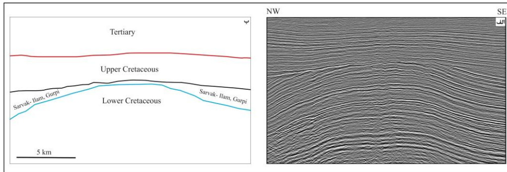
شکل ۴: الف) مقطع لرزه‌نگاری بازتابی عمود بر تاقدیس تنگو. ب) تفسیر زمین‌شناسی این مقطع بازتابی. ناپیوستگی کرتاسه بالایی که سبب حذف یا کاهش ضخامت رسوبات شده است، تجدید فعالیت گسل هندوچان در کرتاسه بالایی را نشان می‌دهد.
