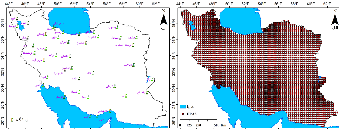
شکل ۱: منطقه مورد پژوهش و پراکنش فضایی داده‌های مورد بررسی: الف: موقعیت مکانی یاخته‌های شبکه‌ای ERA5 (قدرت تفکیک ۰/۲۵×۰/۲۵) و ب: موقعیت مکانی ایستگاه‌های همدید استفاده شده برای ارزیابی شبکه‌ای ERA5
