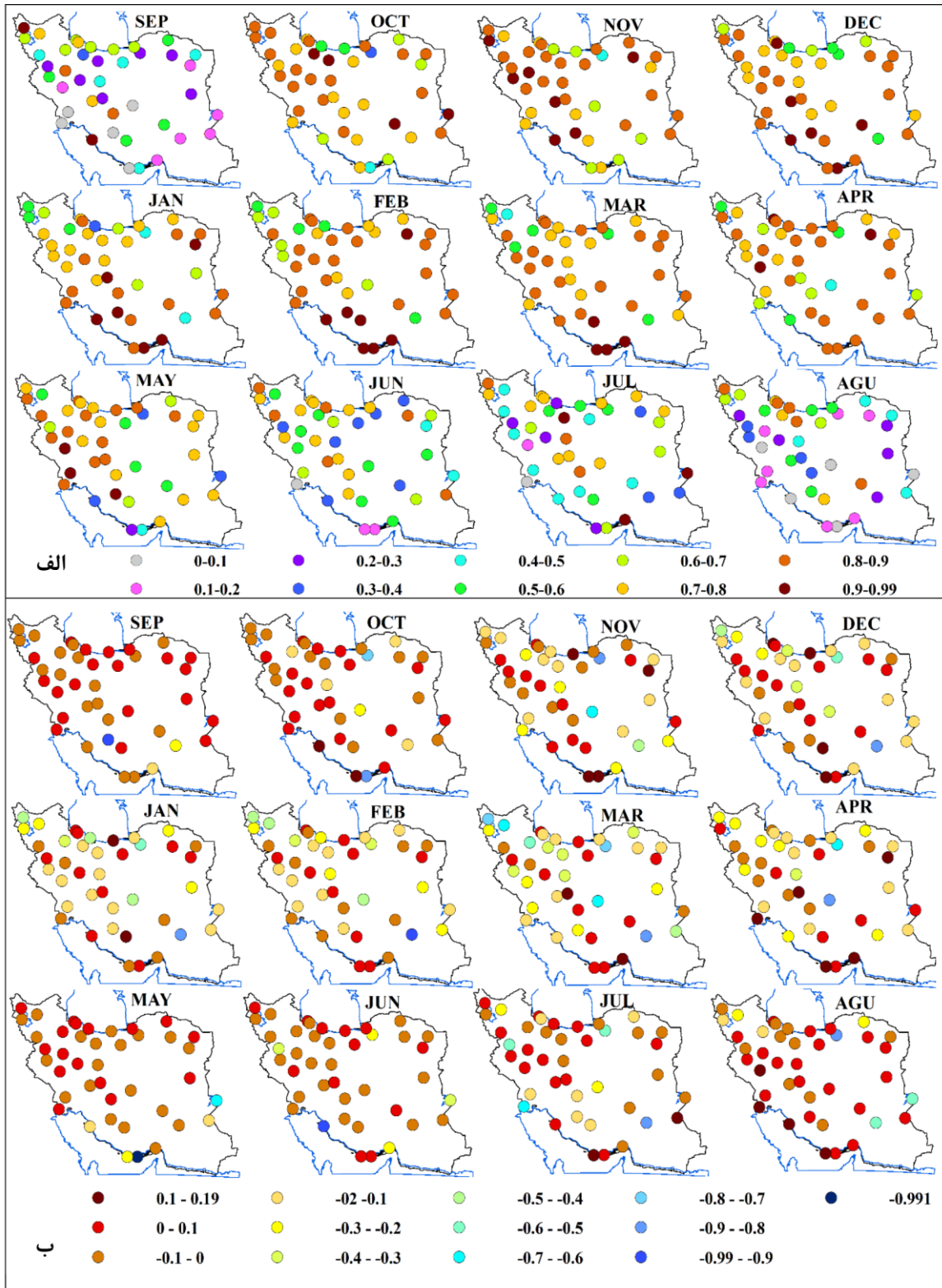
شکل ۴: بخش الف: شاخص توافقی ویلموت، بین بارش ماهانه (میلی‌متر) در نزدیک‌ترین یاخته در شبکه داده ERA5 نسبت به بارش ماهانه ایستگاه همدید می‌باشد. بخش ب: شاخص آریبی استاندارد شده (Standard BIAS) بین بارش ماهانه (میلی‌متر) در نزدیک‌ترین یاخته در شبکه داده ERA5 نسبت به بارش ماهانه ایستگاه همدید می‌باشد، در این ضریب بایاس استاندارد منفی (بیش برآوردی) و بایاس استاندارد مثبت (کم برآوردی) می‌باشد.
