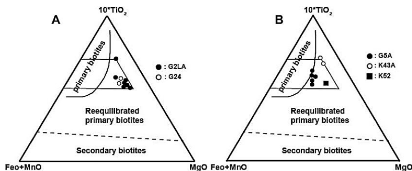
شکل ۵: نمودار مثلثی 10^*TiO_2-MgO-FeO+MnO برگرفته از نچیت و همکاران (۲۰۰۵) جهت تعیین اولیه و یا ثانویه بودن بیوتیت‌ها و موقعیت بیوتیت‌های آتشفشان سارای بر روی آن.
