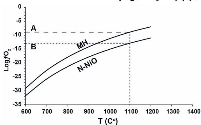
شکل ۱۰: نمودار T-LogfO 2 و نمایش واکنش‌های بافر HM و Ni-NiO بیوتیت‌های آتشفشان سارای در این نمودار
