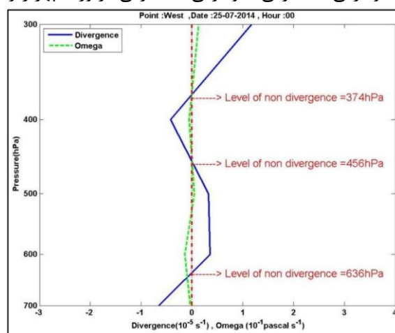
شکل ۱۳: نیمرخ قائم واگرایی (خط ممتد آبی) و امگا (خط چین‌های سبز) در غرب ایران در ساعت ۰۰:۰۰ گرینویچ روز بیست و پنجم ژوئای سال ۲۰۱۴. همگرایی - واگرایی - همگرایی - واگرایی در وردسپهر زیرین، میانی، میانی و بالا.
