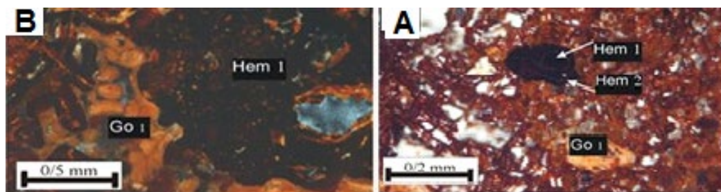
شکل ۵: تصاویر میکروسکوپی از مقاطع صیقلی. (A) بلورهای هماتیت نسل اول که توسط گوتیت و هماتیت‌های نسل دوم جانشین شده‌اند. (B) گوتیت با بافت کلوفرم و جانیشینی (XPL). (Hem: هماتیت، Go: گوتیت).
