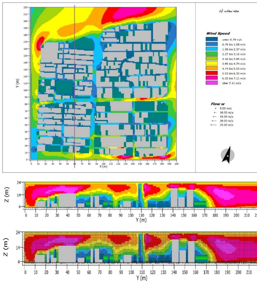
شکل ۸: بردارهای باد در محله سعادت‌آباد در مقطع Y-Z (Y=55)
