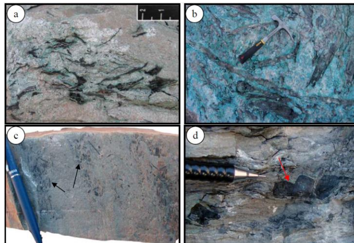
شکل ۶: نمایی از قطعات فسیل‌گیاهی و اشکال مختلف آن. (a و b) قطعات بزرگ فسیل‌گیاهی که در بخش‌های با نفوذپذیری بالا قرار دارند. طول برخی از این فسیل‌ها به بیشتر از یک متر می‌رسد. (c) فسیل‌های ریز که در بخش‌های نفوذناپذیر قرار داشته و کانه‌زایی در آنها دیده نمی‌شود. (d) قطعات گردشده فسیل‌های گیاهی.
