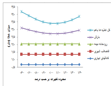
حساسیت مدل نسبت به مقادیر تغذیه
