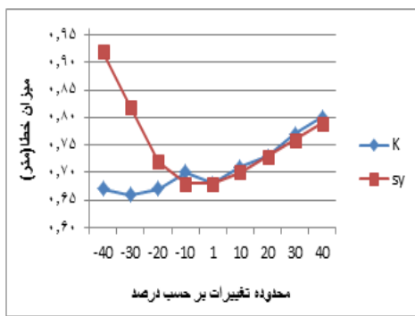
حساسیت پارامترهای K و Sy در مدل گستره مورد مطالعه
