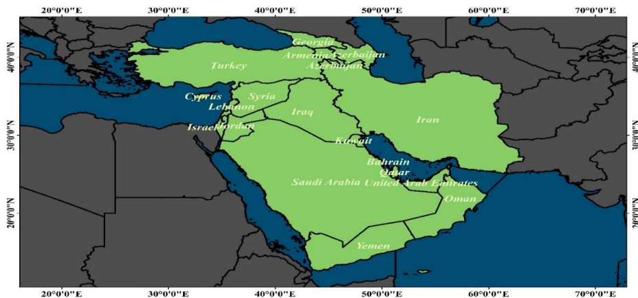
شکل ۱: منطقه مورد مطالعه (غرب آسیا)
