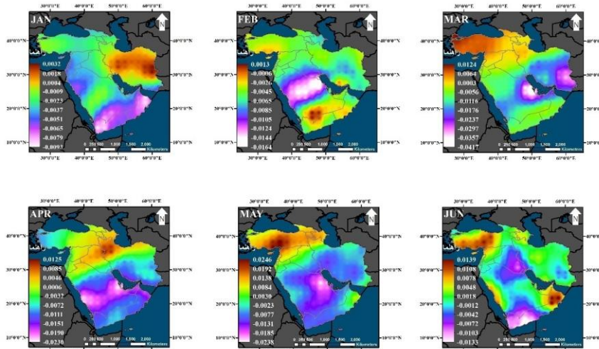
شکل ۴: بی‌هنجاری عمق نوری هواویز براساس سناریوی SSP1-2.6 در فصل‌های زمستان و بهار در آینده نزدیک (۲۰۲۱-۲۰۶۰).
