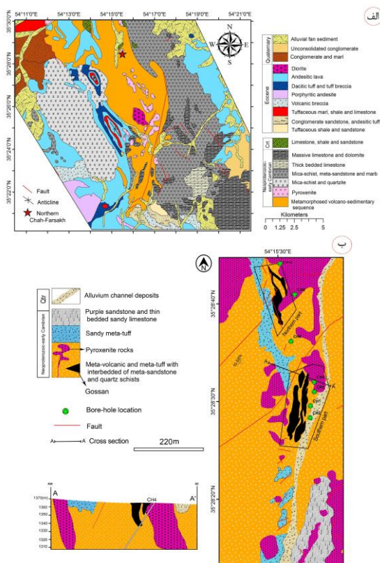
شکل ۲: الف: نقشه زمین‌شناسی ساده شده ۱:۱۰۰,۰۰۰ کلاتهرشم و موقعیت کانسار چاه فرسخ شمالی در توالی آتشفشانی-رسوبی دگرگون شده نئوپروتروزوئیک-کامبرین زیرین (با تغییرات از جعفریان، ۱۳۸۰)، ب: نقشه زمین‌شناسی منطقه معدنی کانسار چاه فرسخ شمالی و جایگاه چینه‌های کانه‌زایی مس در سنگ‌های متاولکانیکی، متاتوف و سنگ‌های شیستی (با تغییرات از حمامی‌پور، ۱۳۹۶).
