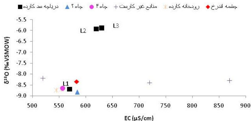
شکل (۸)- نمودار ترکیبی ^{18}\text{O} در مقابل EC نمونه های آب زیرزمینی و سطحی در منطقه
