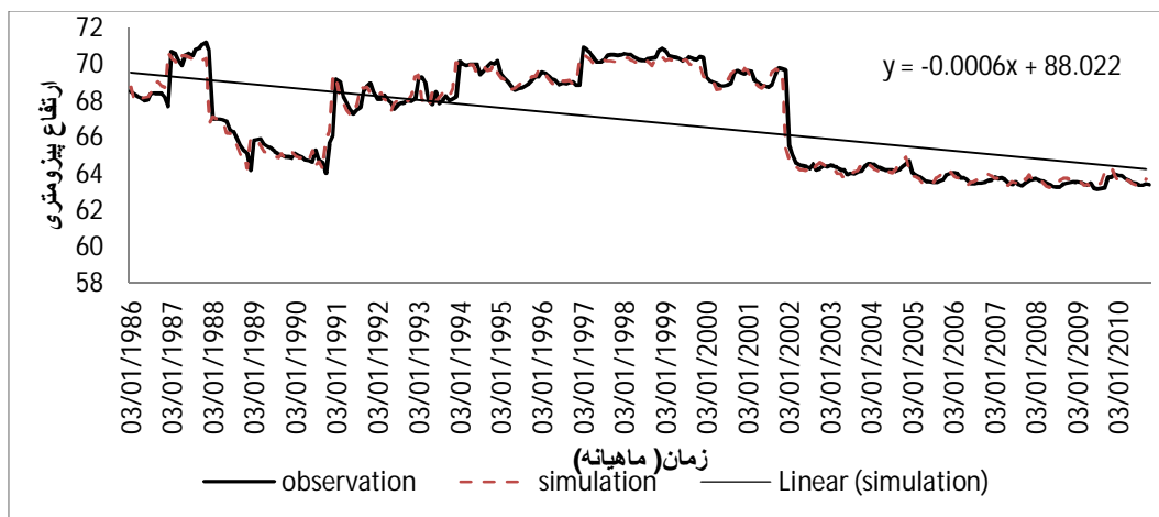
شکل 5: میانگین چند نمونه چاه پیژومتری دور از رودخانه (شبیه سازی شده)
