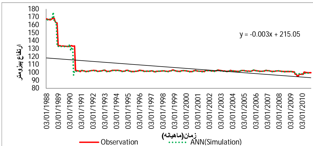
شکل 6: میانگین چندنمونه چاه پیزومتری نزدیک به رودخانه (شبیه سازی شده)
