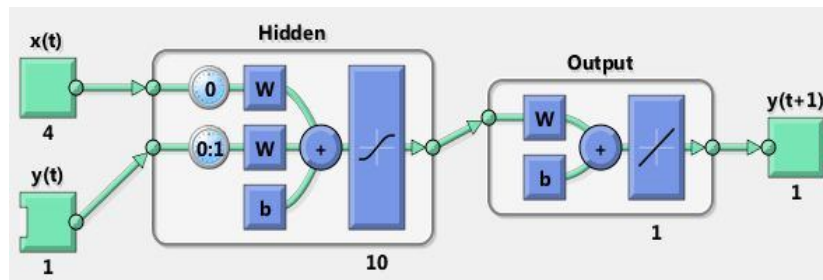
شکل 3: نمایی از پیش بینی شبکه عصبی NARX
