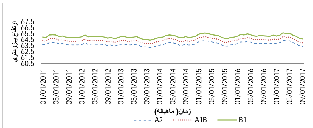
شکل 7: پیش بینی شبکه عصبی پیزومترهای دور از رودخانه
