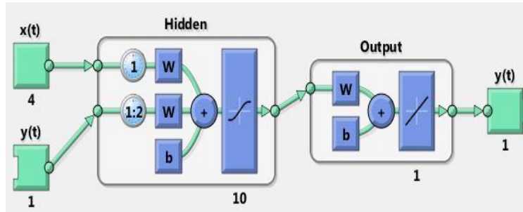
شکل 2: نمایی از شبیه سازی شبکه عصبی NARX
