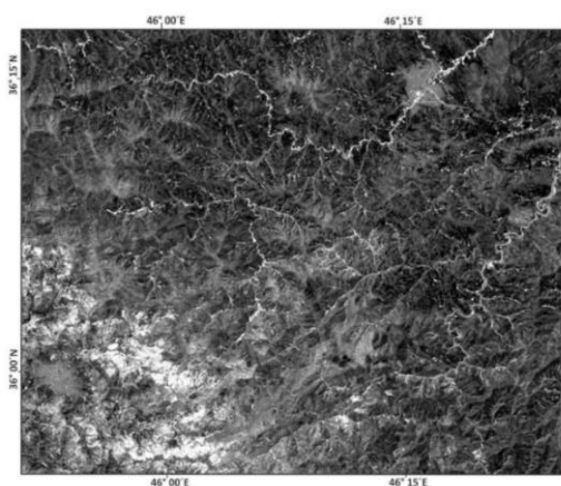
شکل ۱۰: تصویر نسبت باندهای ۳/۴ تصویر ماهواره لندست ۸ برای جدایش راهها که در این تصویر راهها با تن رنگی بالایی نشان داده می‌شوند که به دلیل انعکاس نسبتاً بالا در باند قرمز (TM3) و انعکاس کم در باندهای مادون قرمز میانی (TM7).
