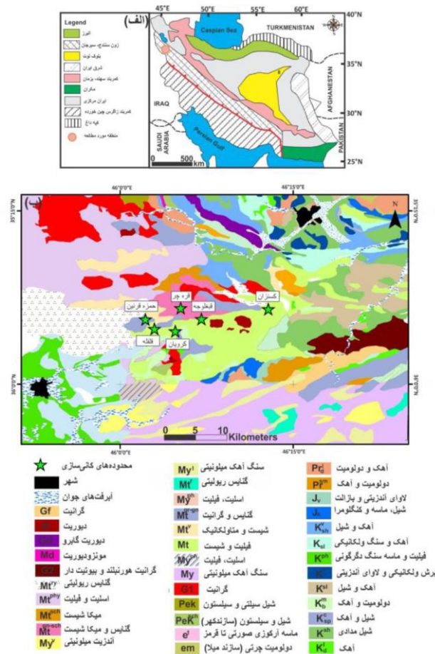
شکل ۱: الف) موقعیت منطقه مورد مطالعه بر روی نقشه ساختاری ایران (Stocklin, 1968)، ب) نقشه زمین‌شناسی ناحیه مورد مطالعه با استفاده از نقشه‌های ۱:۱۰۰۰۰۰ زمین‌شناسی سقز (باباخانی و همکاران، ۱۳۸۲)، آلت (عمرانی و خبازنیا، ۱۳۸۲)، نقشه ۱:۲۵۰۰۰۰ بانه-مریوان (نوگل سادات و هوشمندزاده، ۱۳۷۲).
