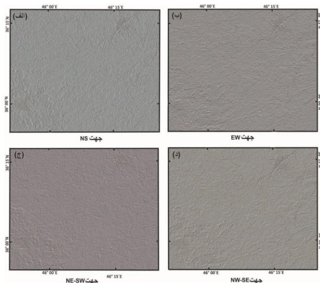
شکل ۳: تصویرهای فیلتر شده با فیلتر جهت‌دار Prewitt که روند خطواره‌ها در چهار راستای الف) شمالی- جنوبی (NS)، ب) شرقی- غربی (EW)، شمال شرقی- جنوب غربی (NE-SW) و شمال شرقی- جنوب غربی (NW-SE) را نشان می‌دهد.
